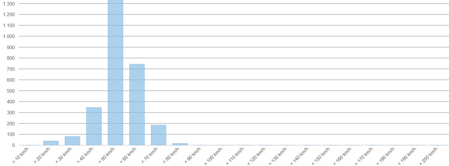
Anzahl Messwerte über Geschwindigkeitsintervall
